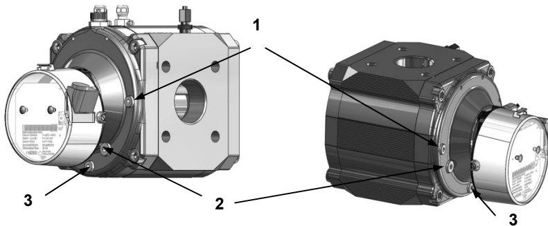
1 = Маслонаполнительный патрубок 2 = Масломерный патрубок 3 = Маслоспускной патрубок
